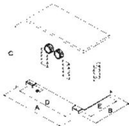
Dimensiones (mm)
